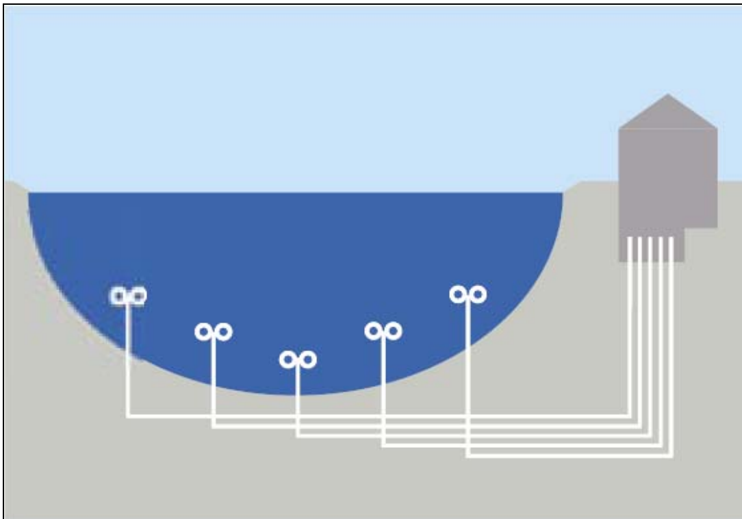
Abbildung 29: Querschnittsprofil der Rheinüberwachungsstation in Weil am Rhein mit schematischer Anordnung der 5 Probenstränge (Kunststoff und Stahl).
