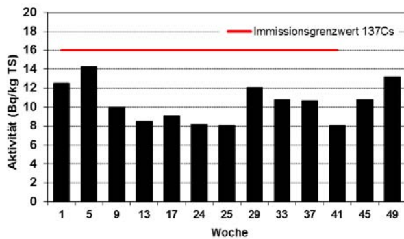
137 Cäsium
