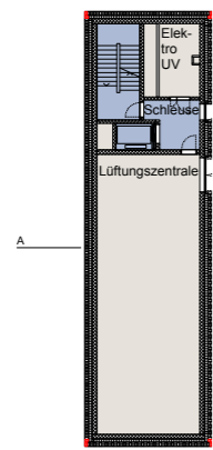
5. OG
