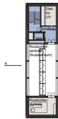
7. OG
