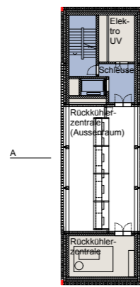
6. OG
