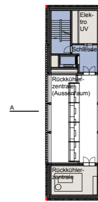
8. OG
