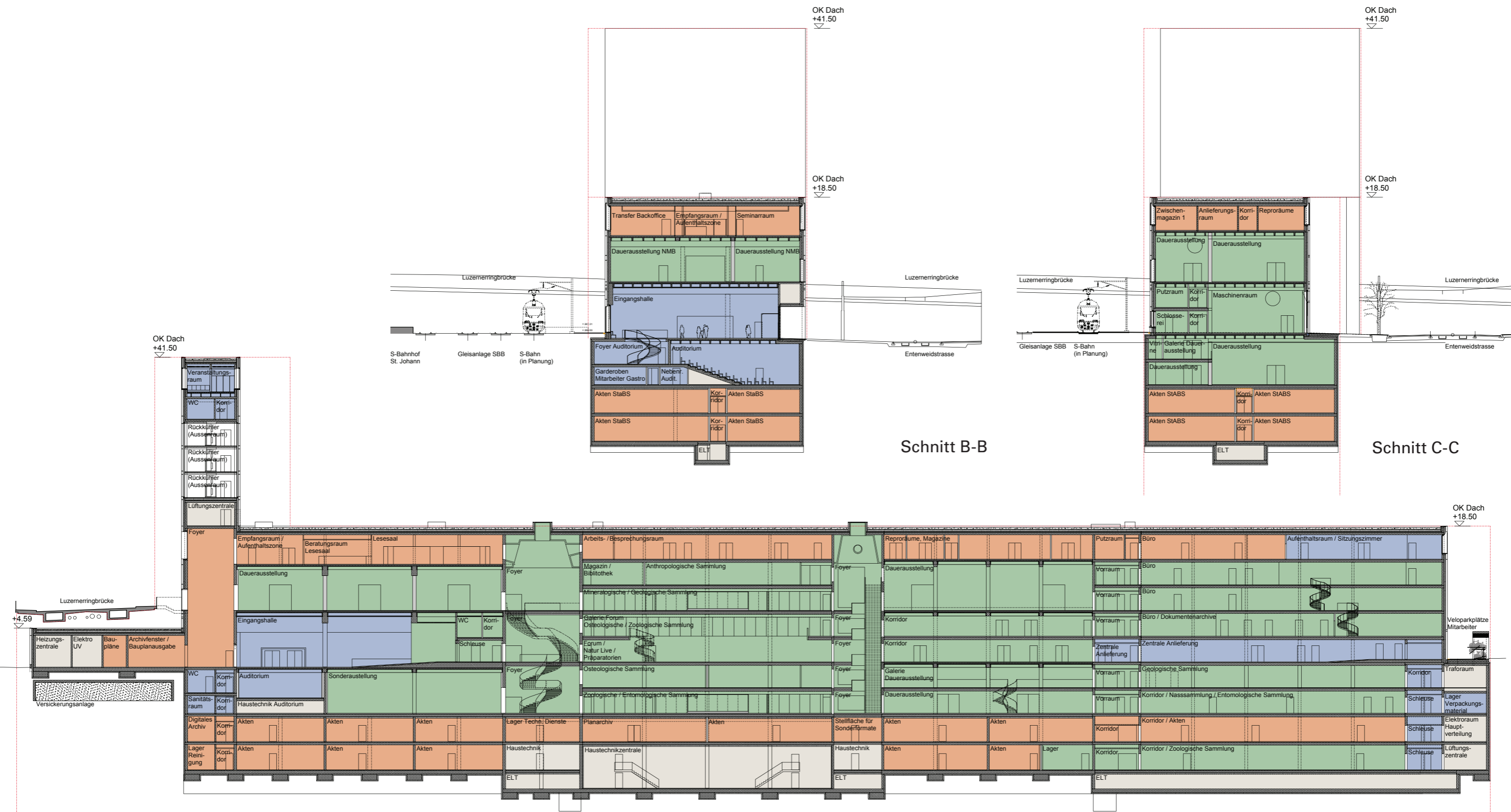
Schnitt A-A
