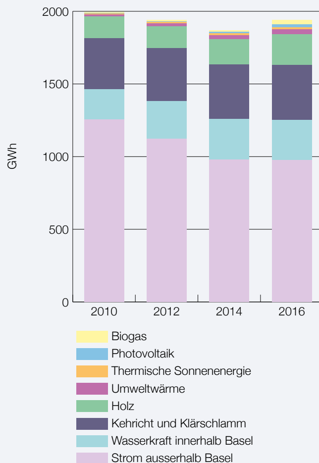
Abbildung 8 Erneuerbare Energien pro Energieträger (Basis Bruttoenergie)
