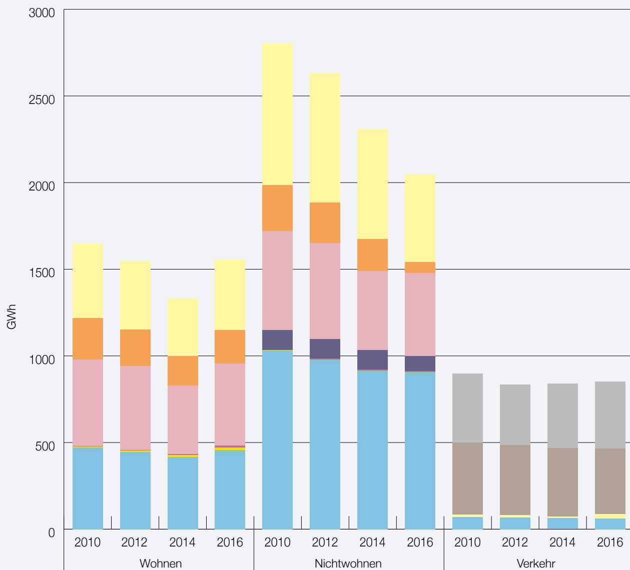
Abbildung 4 Energieverbrauch pro Energieträger und Verbrauchergruppe in den Jahren 2010 bis 2016 (Basis Endenergie)
