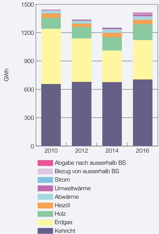
Abbildung 7 Energieeinsatz in der Fernwärme für die Erzeugung der Wärme
