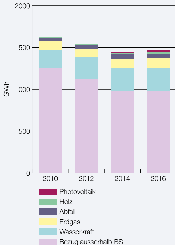
Abbildung 9 Stromerzeugung / Strombezug (Basis Bruttoenergie)
