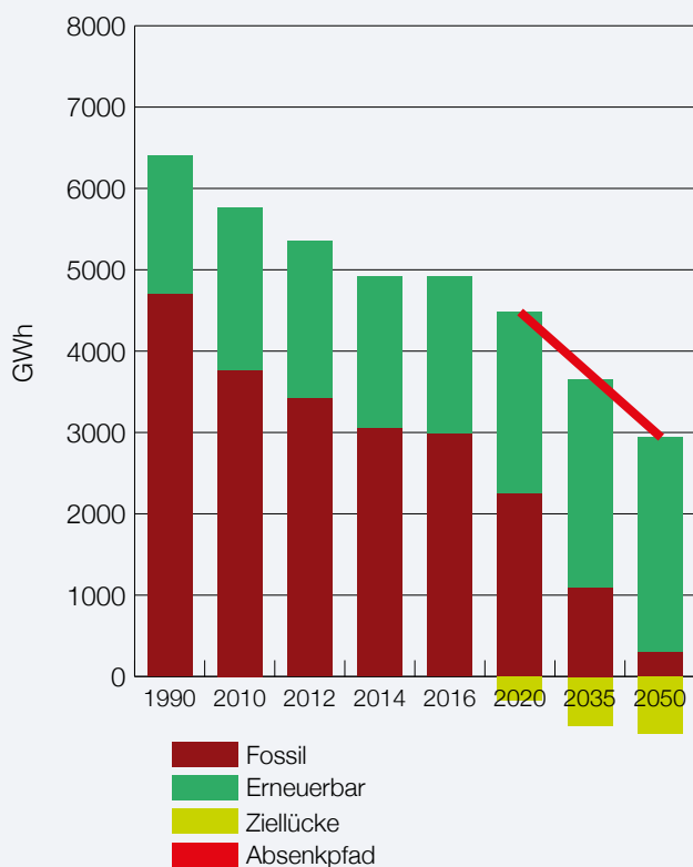
Abbildung 12 Anteil erneuerbar und fossil am Bruttoenergieverbrauch 2010 bis 2016
