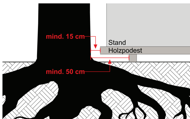
Schematische Darstellung eines Podestbaus zum Wurzel- und Bodenschutz mit Angabe der Minimalabstände zum Baum.
