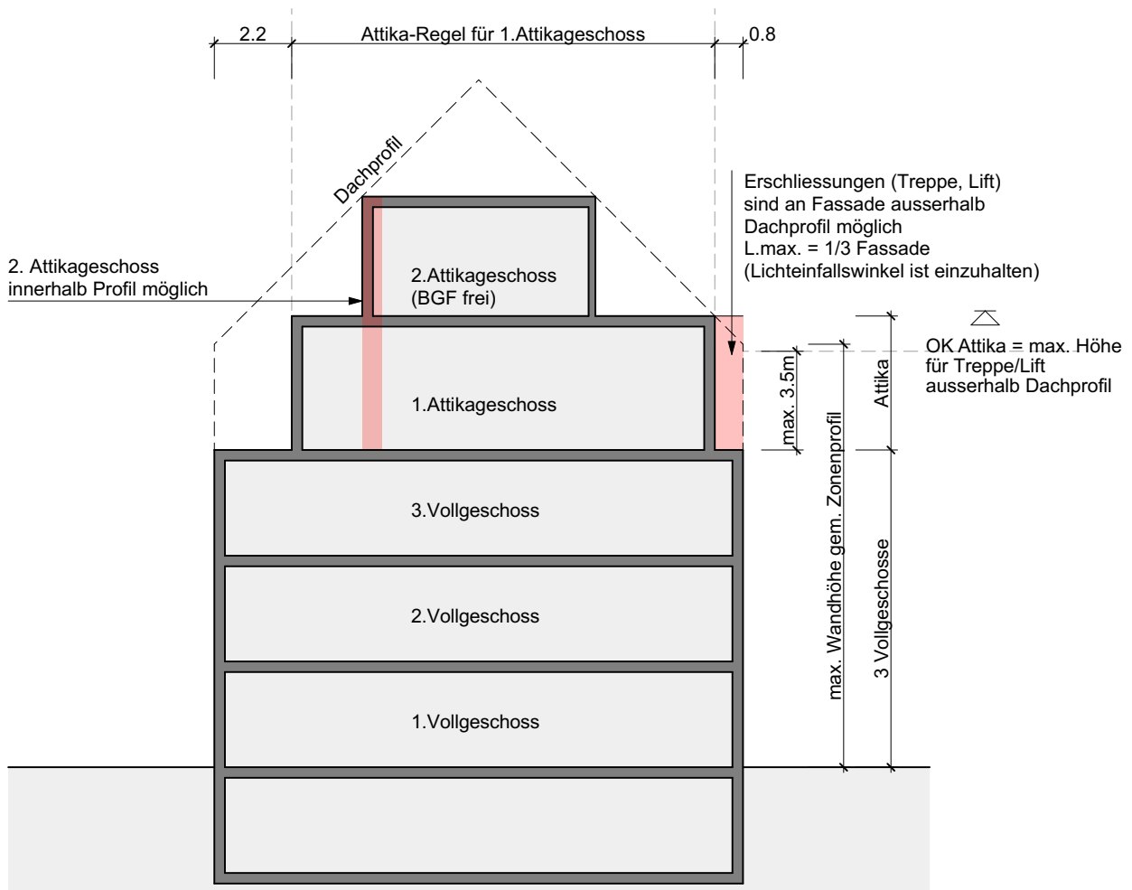
Schema 1 Dachbauvorschriften
