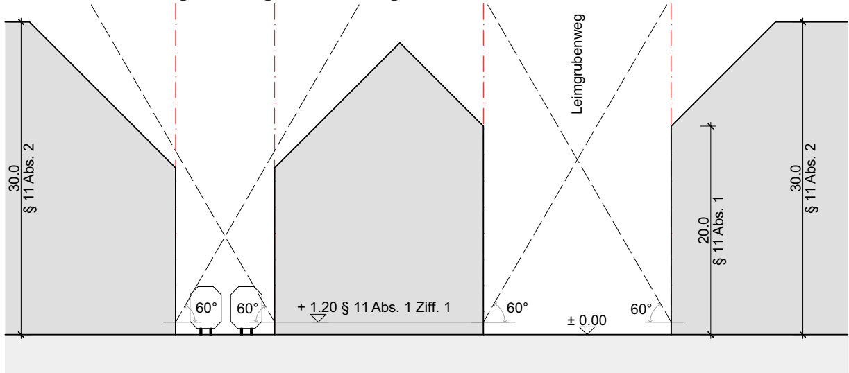
Profil 2: Bauten am Leimgrubenweg und 2-Geleisiger Zufahrt
