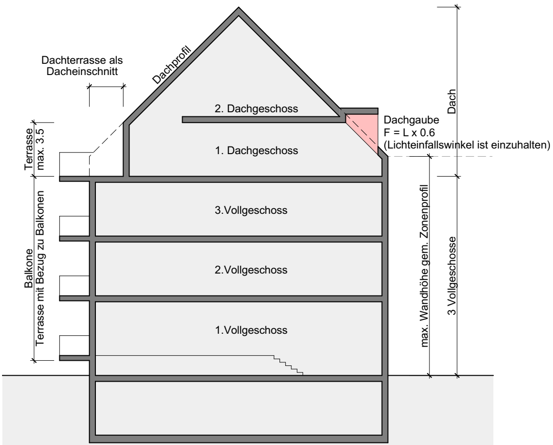
Schema 3 Dachbauvorschriften
