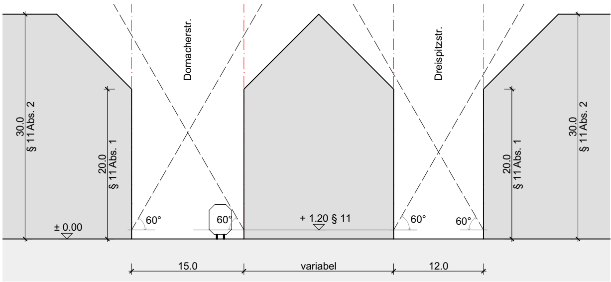
Profil 1: Bauten an der Dornacherstrasse
