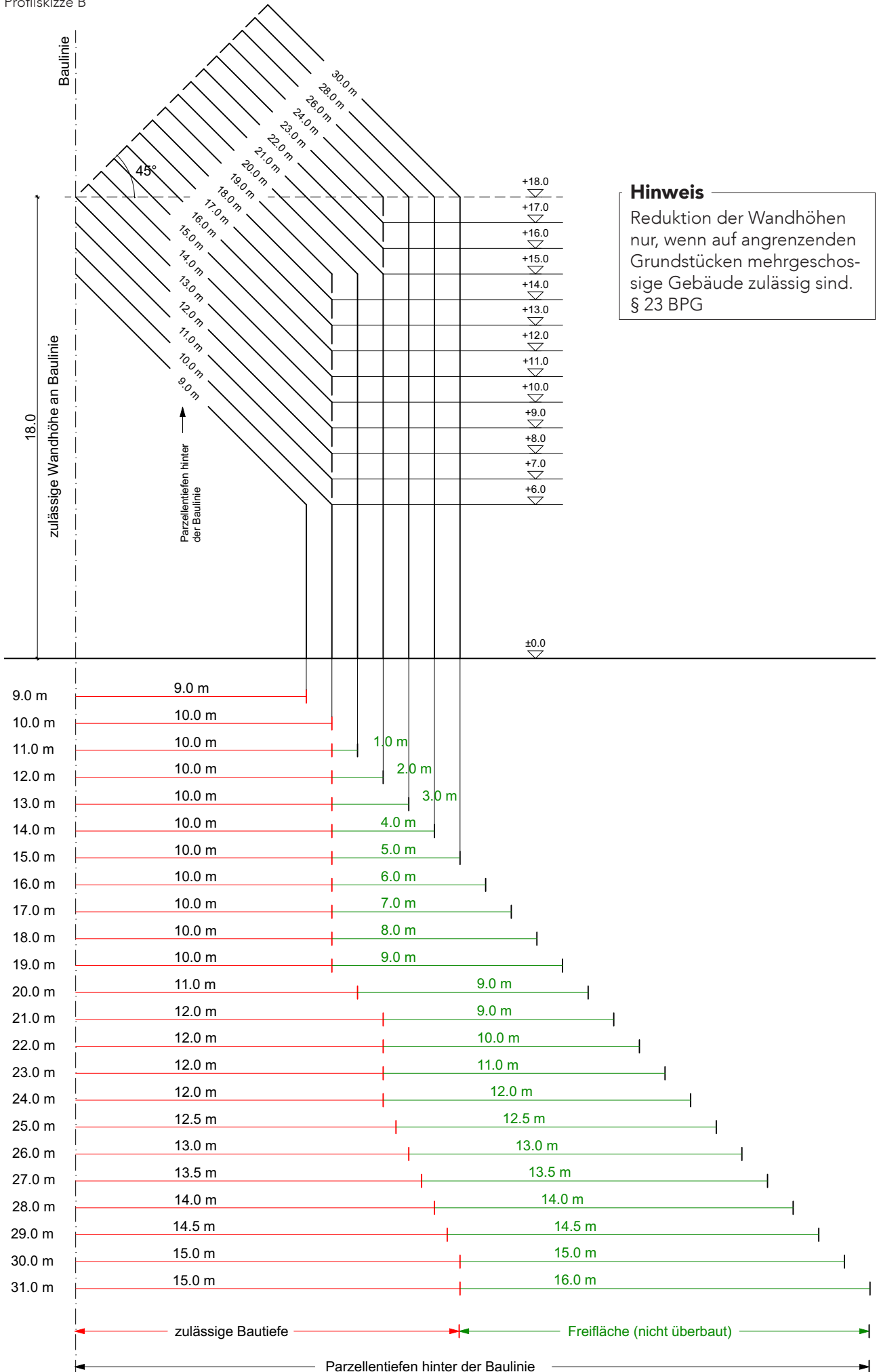
Profilskizze B
