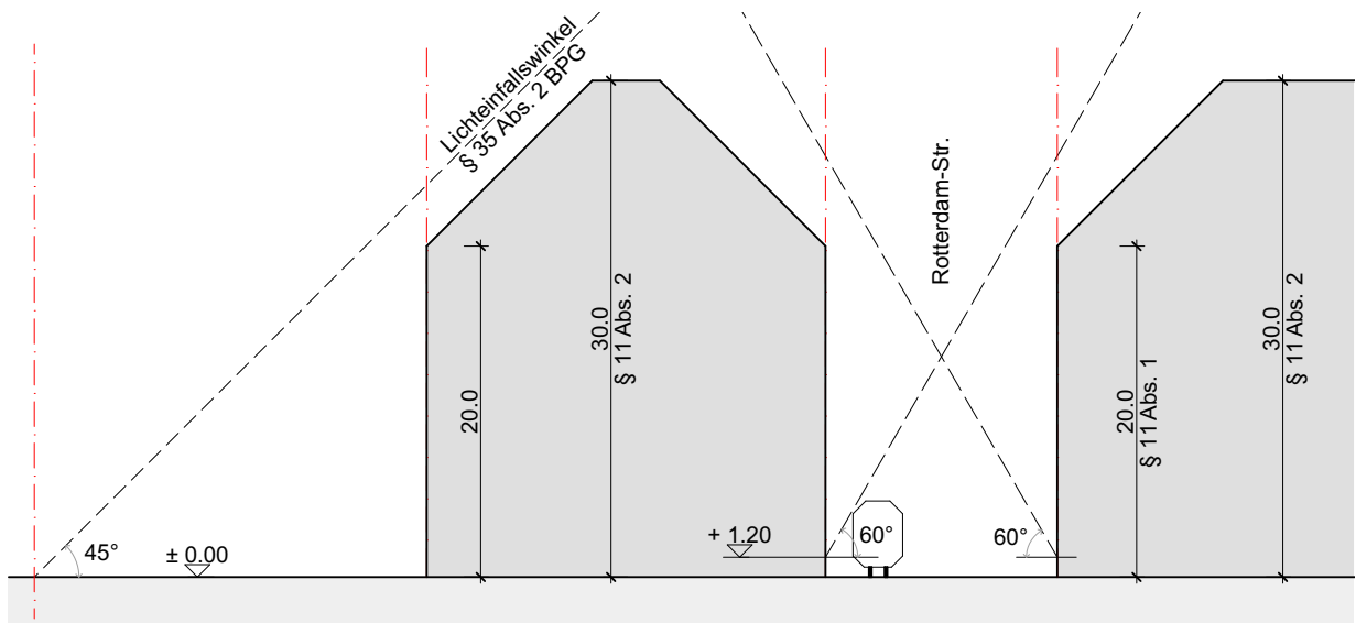
Profil 3: Bauten an der Reinacherstrasse und Münchensteinerstrasse
