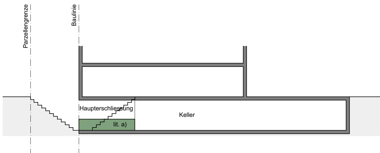
Haupterschließung durch Untergeschoss
