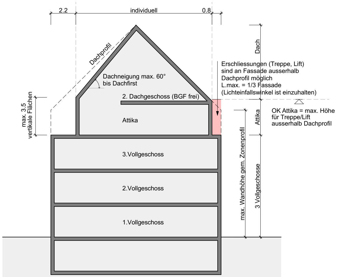
Schema 2 Dachbauvorschriften
