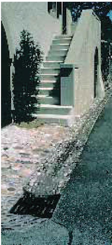
Traditionelle Sammelrinne
