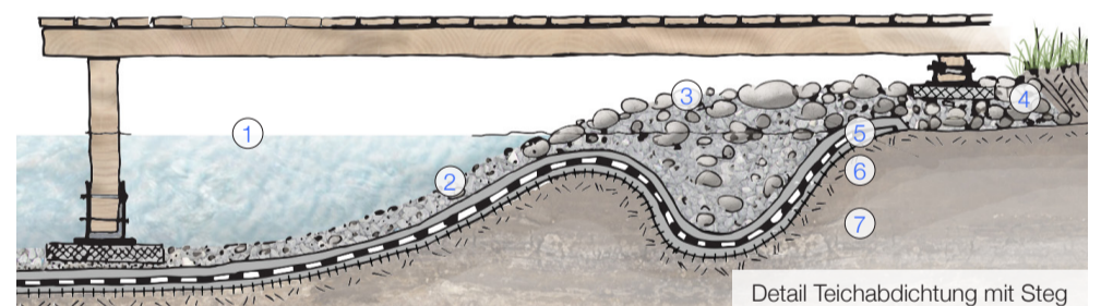
Detail Teichabdichtung mit Steg
