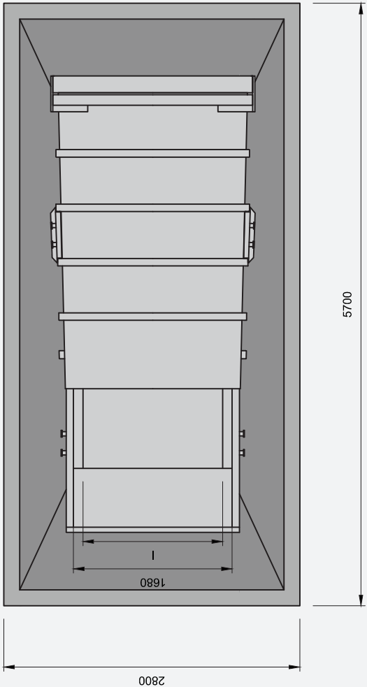
Grundriss
