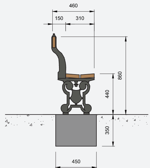
Ansicht quer
