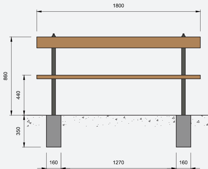
Ansicht längs
