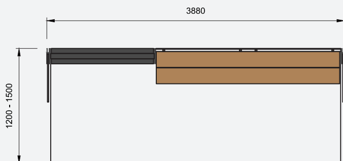
Grundriss
