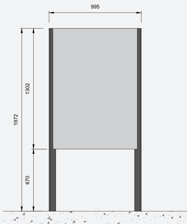
Ansicht längs
