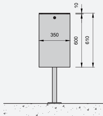
Ansicht quer
