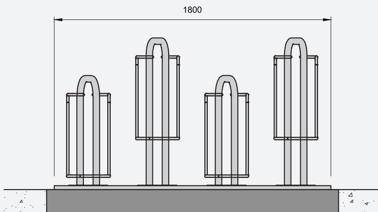
Ansicht längs
