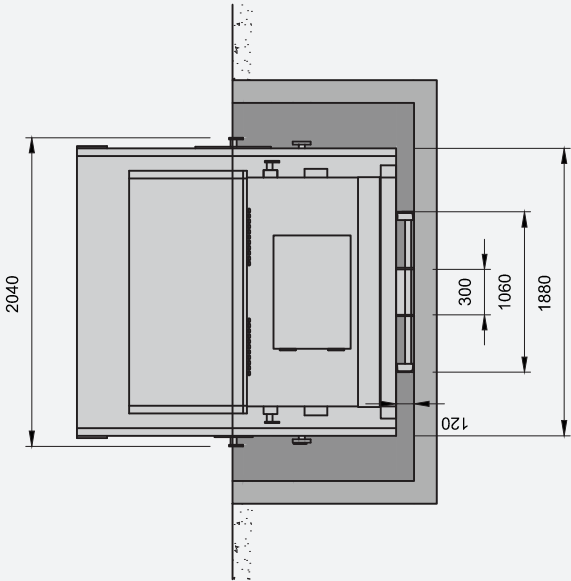
Ansicht quer
