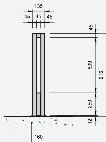
Schnitt quer
