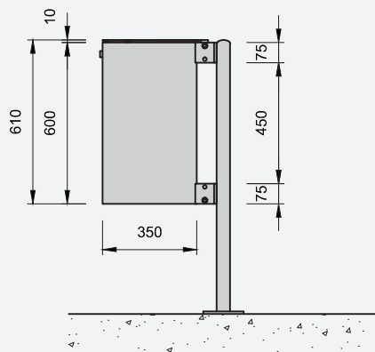
Ansicht längs
