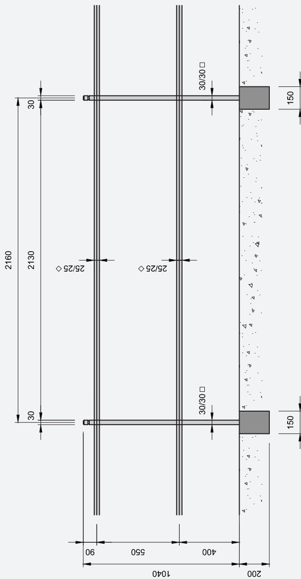
Ansicht längs
