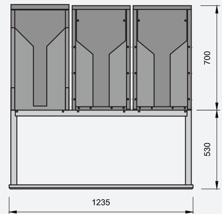
Ansicht längs
