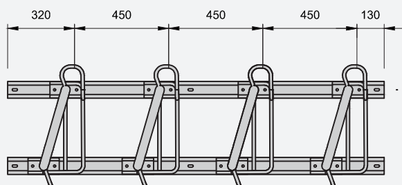
Grundriss
