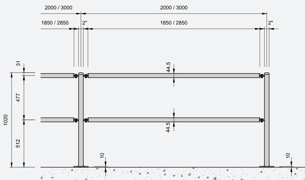
Ansicht längs
