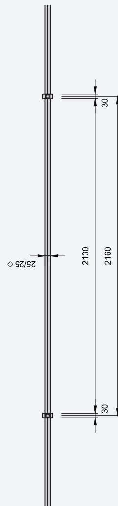
Grundriss
