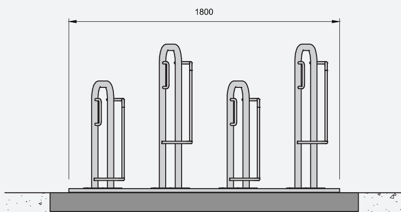
Ansicht längs
