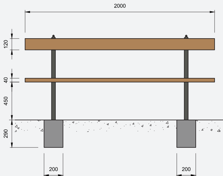
Ansicht längs
