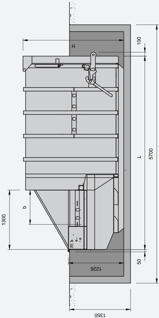
Ansicht längs
