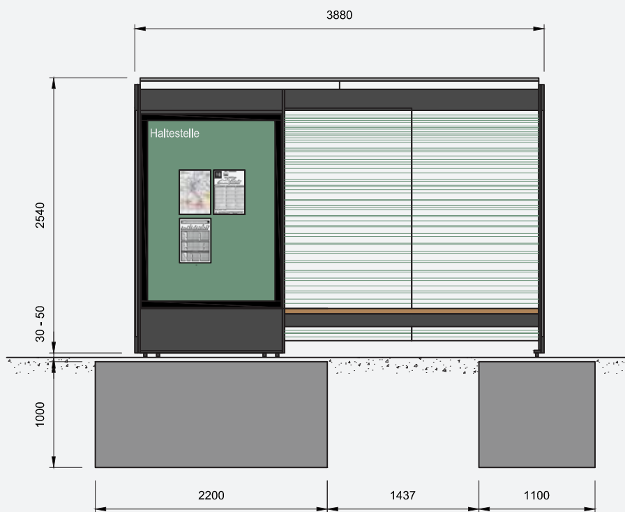
Ansicht längs
