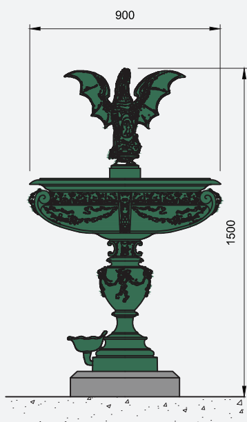
Ansicht längs
