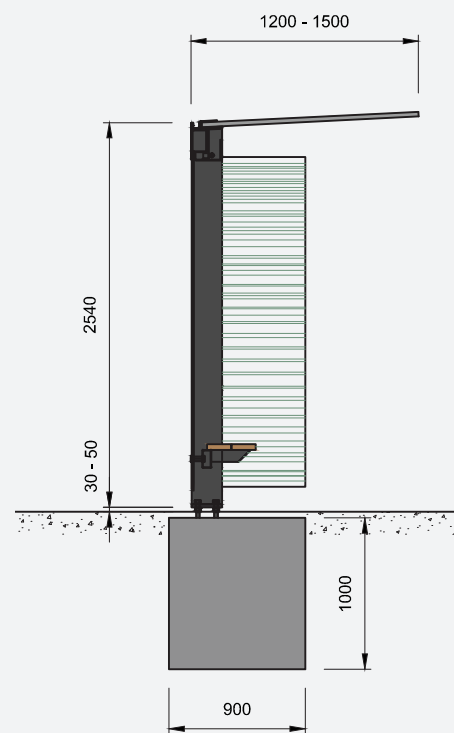
Ansicht quer
