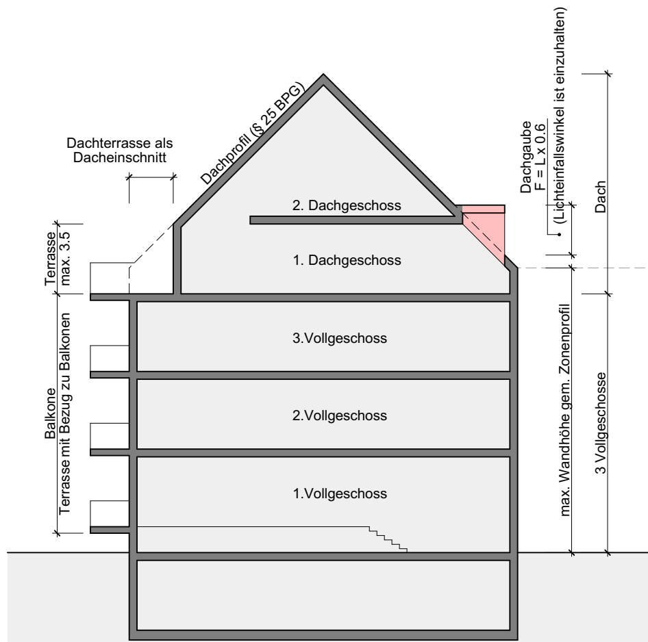
Schema 3 Dachbauvorschriften
