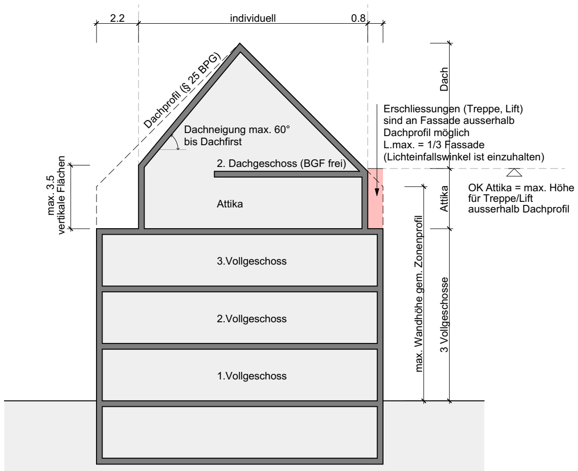
Schema 2 Dachbauvorschriften
