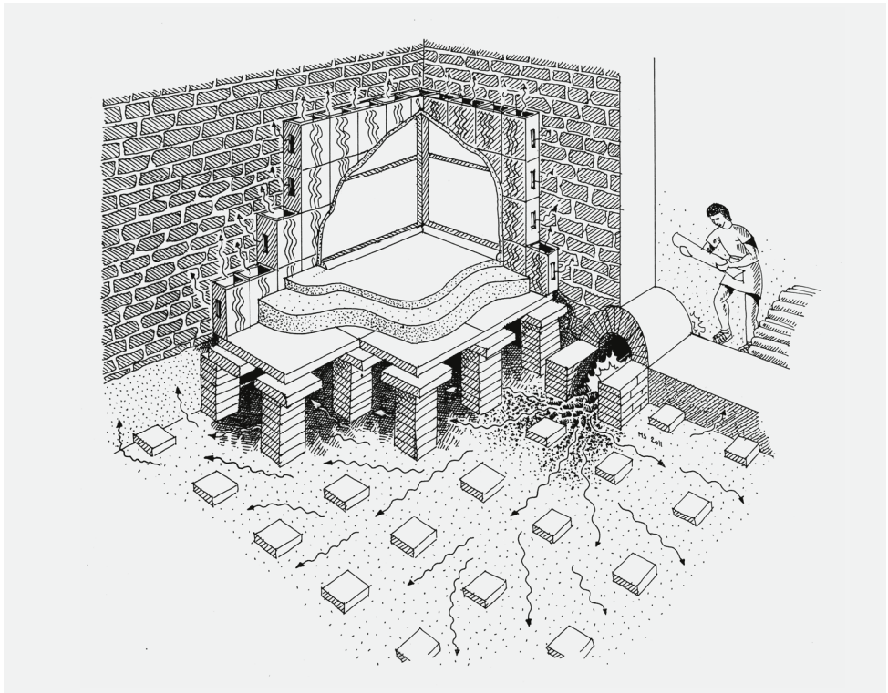
Bei einer römischen Fussbodenheizung strömt die warme Luft unter dem Boden durch und entlang der Wände hoch.
