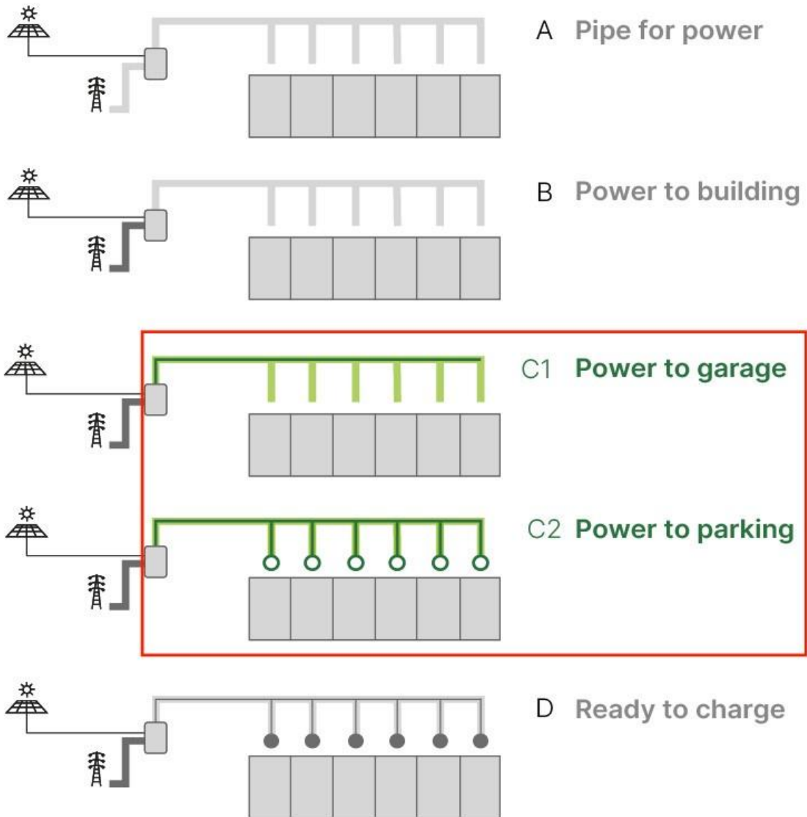
Abbildung 1: Ausbaustufen einer Ladeinfrastruktur nach SIA 2060. Geförderte Ausbaustufen rot umrandet.
