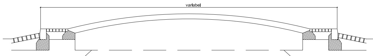
Abb. 204.03b Querschnitt gesamter Kreiselschnitt
