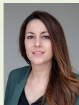
Veronica Gaiardo
